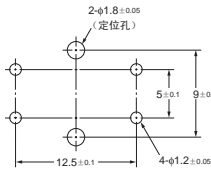
印刷基板孔加工尺寸示例 (TOP VIEW) (单面基板t=1.6)
