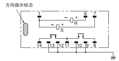
端子配置/内部连接图 (BOTTOM VIEW)
