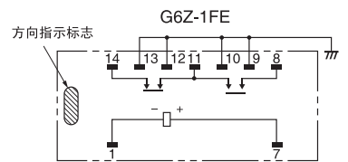
端子配置/内部连接图 (TOP VIEW)
