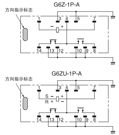
端子配置/内部连接图 (BOTTOM VIEW)
