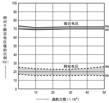
吸合·释放电压的变化
