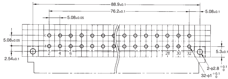
印刷基板加工尺寸 (BOTTOM VIEW)
