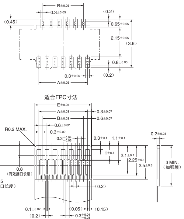
印刷基板加工尺寸 (TOP VIEW)
